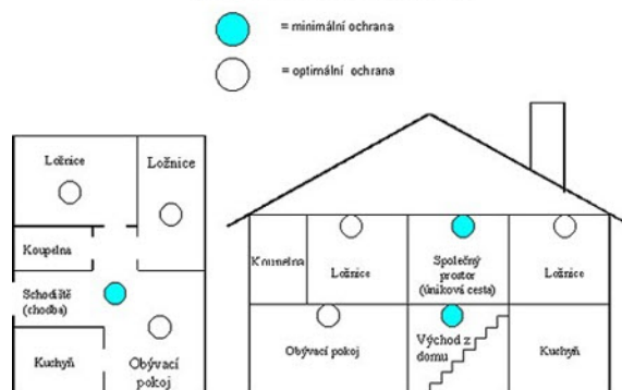
Vhodné rozmístění hlásičů požáru
